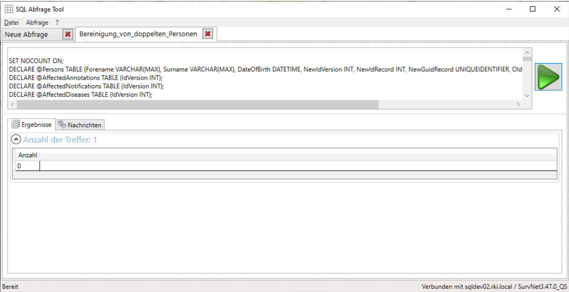
Abbildung 83.15: SQL-Abfrage-Tool
