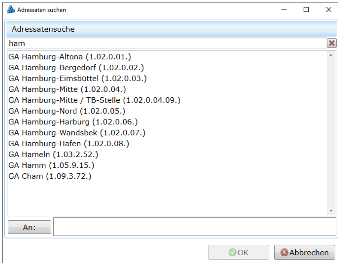
Abbildung 49.1: Fenster Adressatensuche
