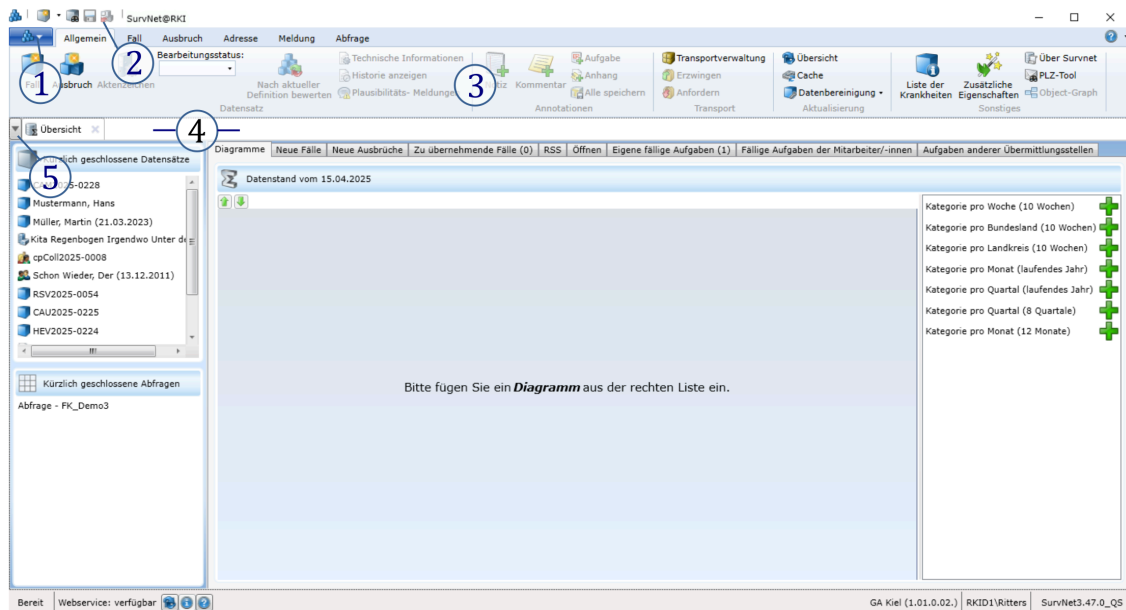
Abbildung 10.1: Die Startansicht
