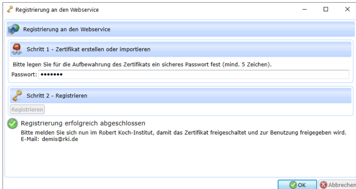
Abbildung 98.1: Webservice-Anmeldung
