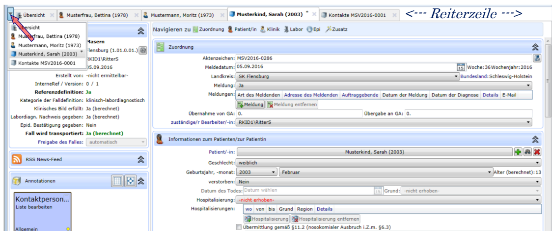
Abbildung 10.10: Die Reiterzeile
