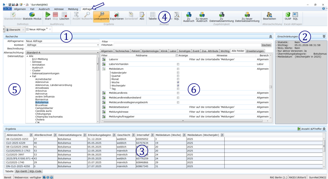
Abbildung 82.1: Das Abfrageformular
