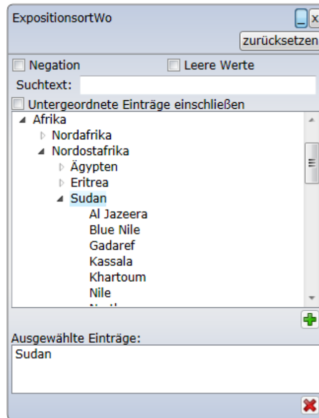
Abbildung 83.2: Listenfeld
