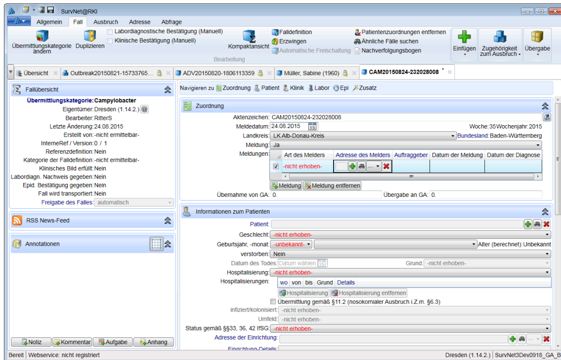
Abbildung 40.1: Auswahlliste
