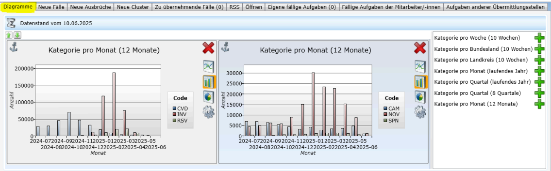
Abbildung 10.2: Diagramme
