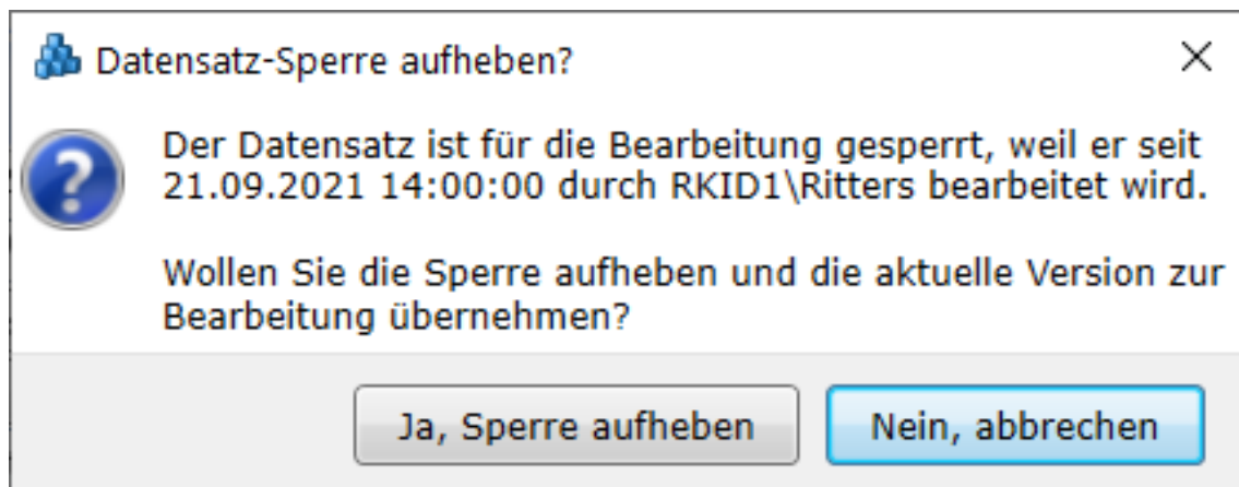
Abbildung 100.5: Notfall-Freigabe
