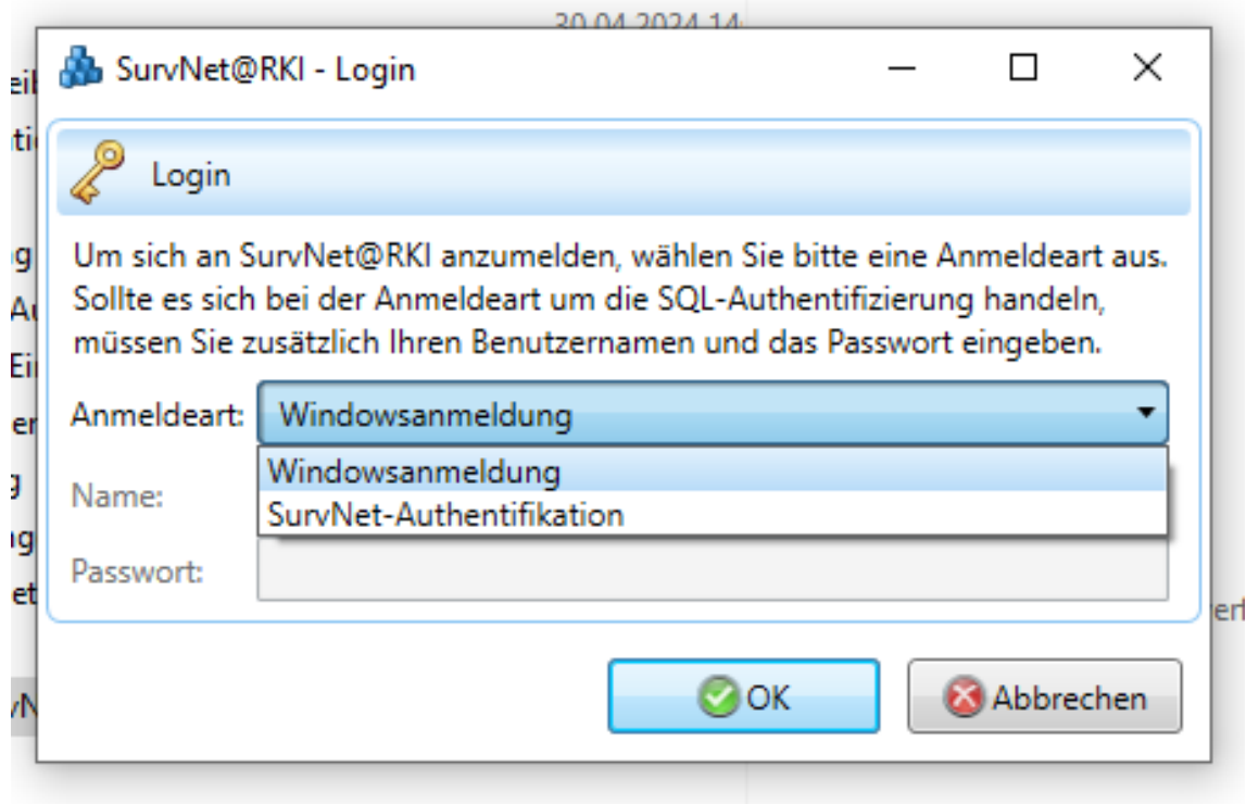
Abbildung 9.1: Login
