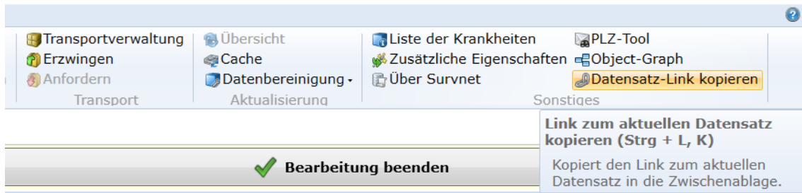
Abbildung 22.1: Datensatz kopieren.
